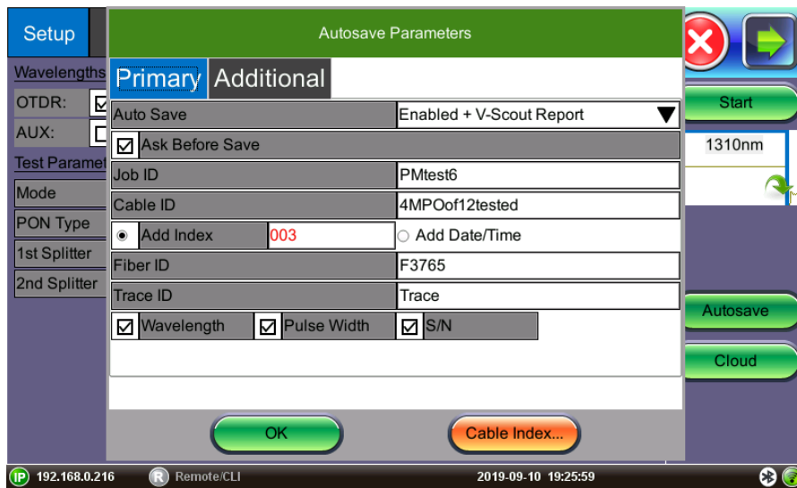
MPO Autosave Parameters
