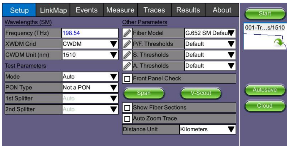
OTDR Setup: RXT-4113 Auto Mode
